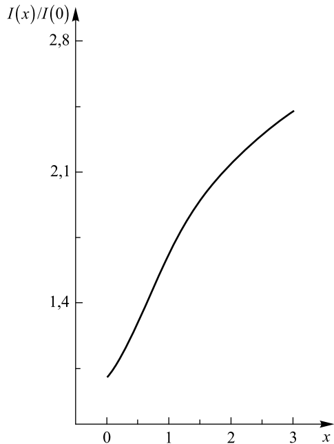
Рис. 3. Зависимость структурных интегралов, определяющих матричный элемент распада S \rightarrow PP , от массы скалярного мезона
