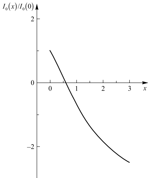
Рис. 3. Зависимость структурных интегралов, определяющих матричный элемент распада S \rightarrow PP , от массы скалярного мезона
