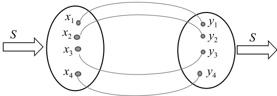
Рис. 7. Массовый оператор мезона в четырехкварковой схеме
