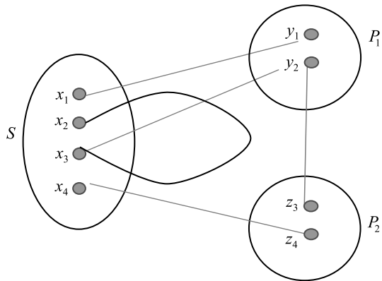
Рис. 8. Кварковые диаграммы, описывающие распад S \rightarrow PP в четырехкварковой схеме
