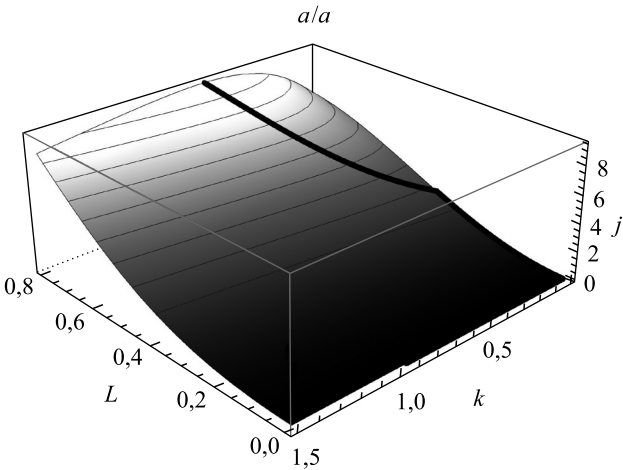
Рис. 7. Зависимость амплитуды переменной составляющей тока j от параметров k и L для S = 0 (а) и S = 0,3 (б)
