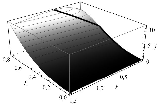
Рис. 7. Зависимость амплитуды переменной составляющей тока j от параметров k и L для S = 0 (а) и S = 0,3 (б)
