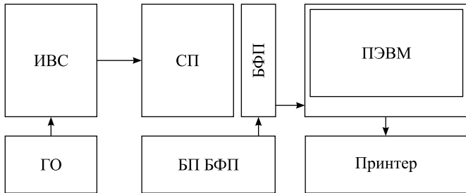
Рис. 1. Блок-схема разработанного и изготовленного спектрометра многоканального атомно-эмиссионного с CLR-генератором MS-200УН
