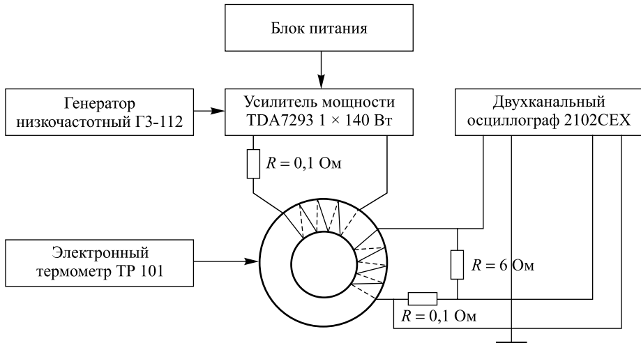
Рис. 1. Схема исследования динамических свойств композиционных магнитно-мягких материалов
