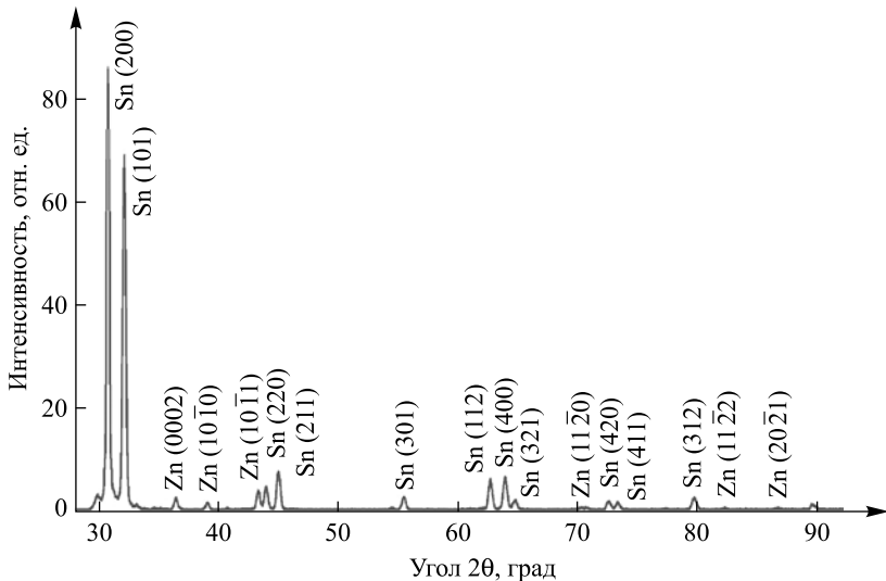
Рис. 1. Рентгенограмма быстрозатвердевшей фольги сплава Sn – 8,8 мас. % Zn
