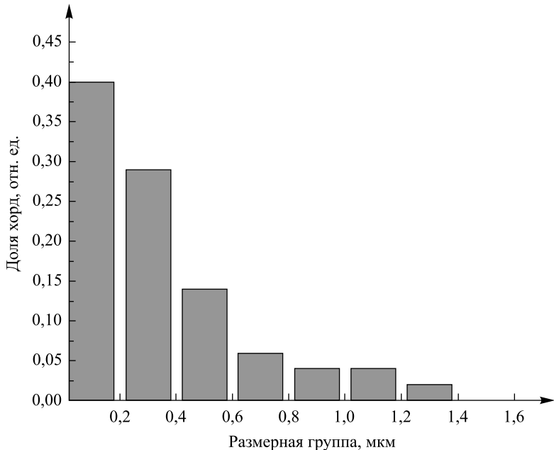
Рис. 3. Распределение хорд случайных секущих на сечениях выделений твердого раствора цинка
