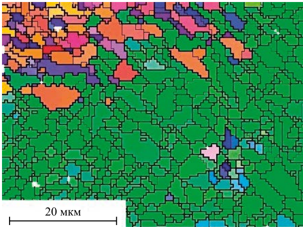
Рис. 4. Зеренная структура твердого раствора олова фольги сплава Sn – 8,8 мас. % Zn
