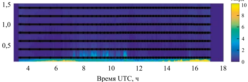
Рис. 2. Вертикальное распределение NO 2 при интенсивном движении автотранспорта (25 августа 2017 г.)
