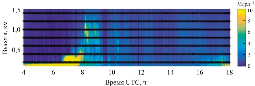
Рис. 3. Вертикальное распределение \text{NO}_2 при конвективном подъеме (10 июня 2017 г.) Fig. 3. \text{NO}_2 vertical profile: upwelling convection (2017 June 10)
