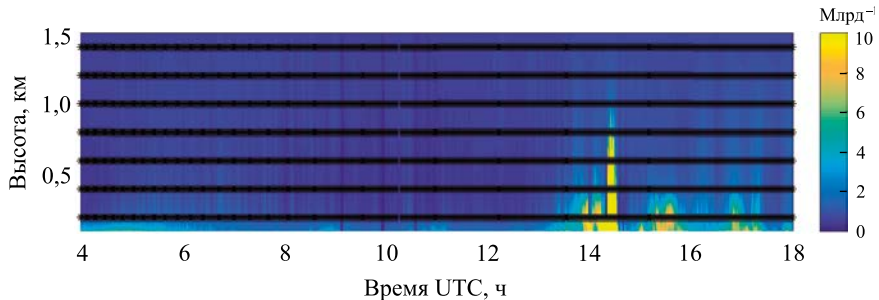
Рис. 4. Вертикальное распределение NO 2 : одиночные всплески (21 июня 2017 г.)
