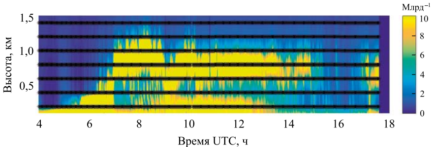
Рис. 5. Вертикальное распределение NO 2 : аномальный случай (19 мая 2017 г.)
