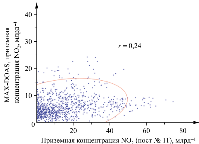
Рис. 9. Сравнение данных о приземной концентрации двуокиси азота в г. Минске (август 2017 г.), полученных методом MAX-DOAS (а, красные точки) и импактным методом отбора проб с использованием газоанализатора (а, черные точки), и корреляционное поле (б)
