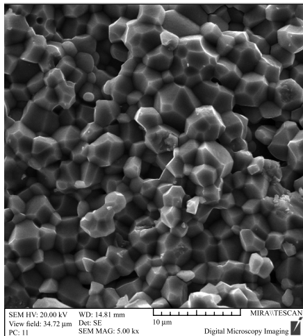
Рис. 3. Микроструктура керамики (спекание: 1700 °С, 1 ч 20 мин) на основе диоксида циркония (ДЦИ-5) при увеличении \times 5000 (а) и \times 10\,000 (б)
