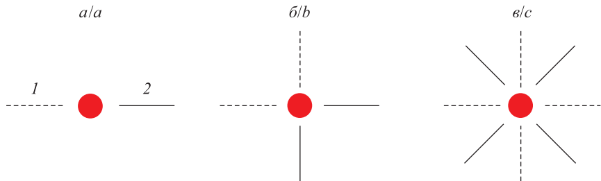
Рис. 2. Схемы пространственных конфигураций электродов: a – парная, b – крестовая, c – восьмиконечная; 1 – катод; 2 – анод
