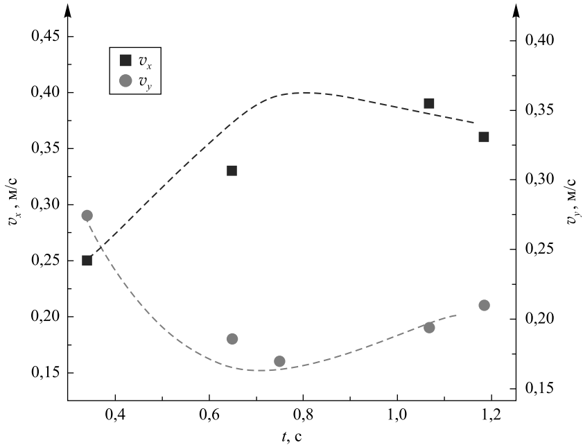
Рис. 4. Зависимость горизонтальной v_x и вертикальной v_y составляющих скорости потока от времени t
