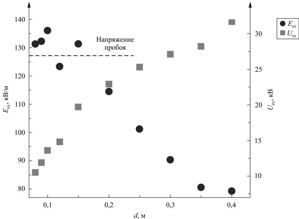
Рис. 6. Зависимость минимального напряжения U_{\text{ex}} и напряженности E_{\text{ex}} ЭП, приводящих к затуханию пламени, от расстояния между электродами d
