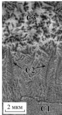
Рис. 2. Микроструктура поперечного сечения фольги сплава Al – 24,5 ат. % Ge
