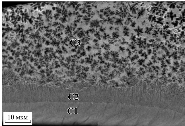
Рис. 2. Микроструктура поперечного сечения фольги сплава Al – 24,5 ат. % Ge
