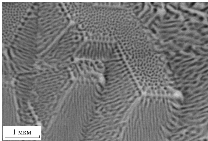
Рис. 3. Микроструктура поперечного сечения (а) и поверхностей А (б) и В (в) фольги сплава Al – 28,2 ат. % Ge Fig. 3. The microstructure of the cross section (a) and surface A (b) and surface B (c) of the alloy foil Al – 28.2 at. % Ge
