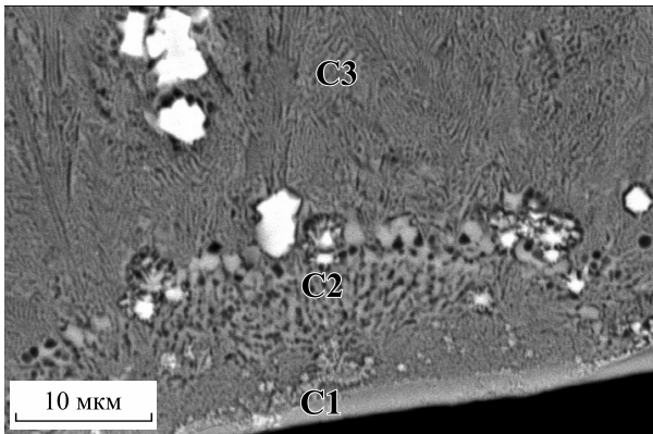
Рис. 4. Микроструктура поперечного сечения фольги сплава Al – 33,3 ат. % Ge
