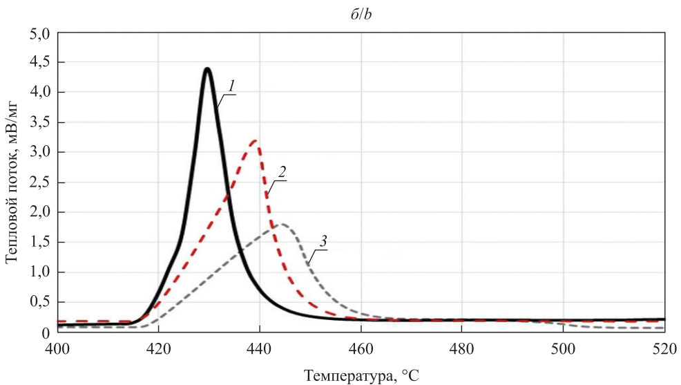
Рис. 5. Термограммы плавления сплавов системы Al – Ge: a – быстрозатвердевшая фольга; b – массивные образцы Fig. 5. Thermograms of melting of alloys of the Al – Ge system: a – rapidly solidified foils; b – massive samples
