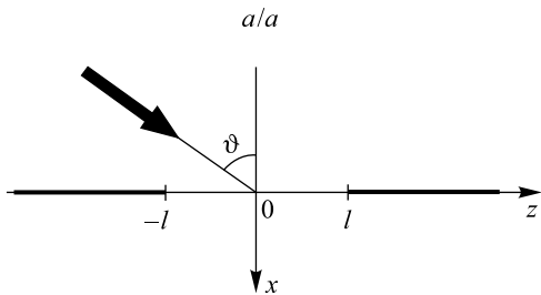
Рис. 4. Дифракция плоской волны на щели в тонком плоском экране ( a ) и на тонкой полосе ( б ): l – полуширина щели (полосы); \vartheta – угол падения волны на плоскость экрана (полосы)
