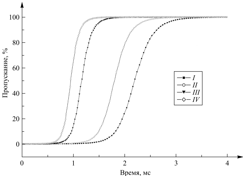
Рис. 3. Времена включения ЖК-ячеек с разной концентрацией НГ: I – НЖК ( t_{\text{БКЛ}} = 0,79 мс); II – НЖК + 0,1 % НГ ( t_{\text{БКЛ}} = 0,65 мс); III – НЖК + 0,5 % НГ ( t_{\text{БКЛ}} = 0,42 мс); IV – НЖК + 1 % НГ ( t_{\text{БКЛ}} = 0,34 мс)
