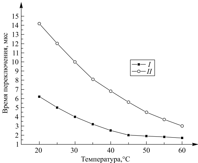
Рис. 6. Время переключения тестовых ячеек:
