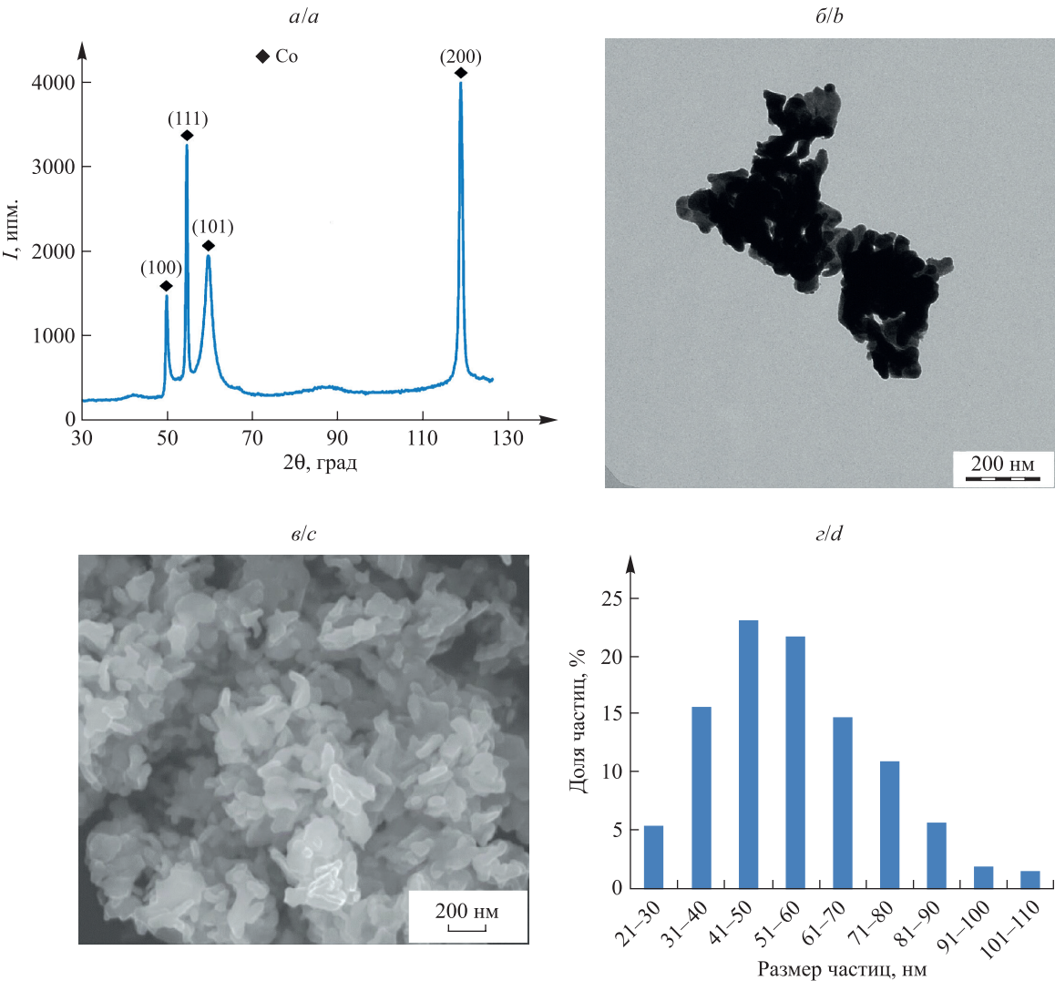
Рис. 5. Рентгенограмма (а), ПЭМ- и СЭМ-изображения (б, в), а также гистограмма распределения по размерам (г) НЧ Co, полученных восстановлением \text{Co}(\text{OH})_2 (с 0,1 % ДСН) при 280 °С в течение 3 ч
