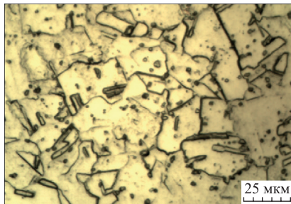
Рис. 3. Структура образца в исходном состоянии ( а ) и после обработки плазмой в течение 5 мин ( б ) и 10 мин ( в ) (прицельная металлография)
