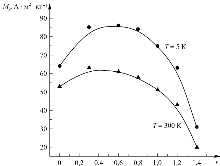
Рис. 3. Зависимость намагниченности насыщения \text{Mn}_x\text{Fe}_{3-x}\text{O}_4 ( 0 < x < 1,4 ) при 5 и 300 К от степени замещения x
