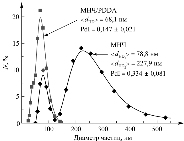
Рис. 4. Распределение по размерам частиц Mn_{0,3}Fe_{2,7}O_4 и Mn_{0,3}Fe_{2,7}O_4/PDDA
