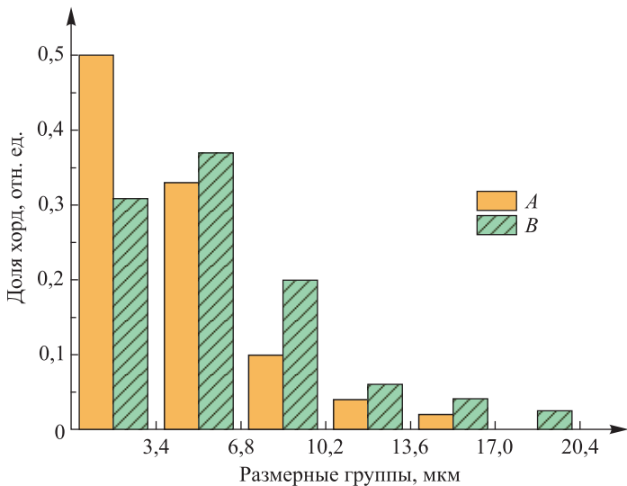
Рис. 3. Распределение хорд случайных секущих на сечениях зерен слоев А и В фольги сплава Sn – 4,4 мас. % Zn
