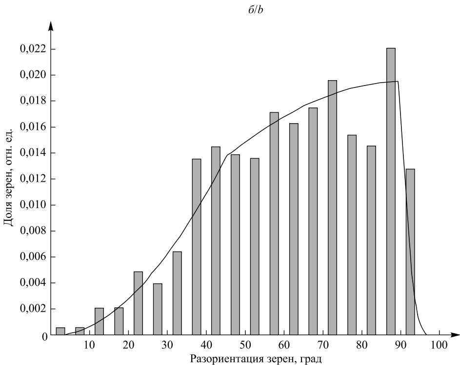
Рис. 5. Разориентация некоррелированных границ соседних зерен в слое, прилегающем к кристаллизатору (а), и в слое, контактирующем с атмосферой (б)
