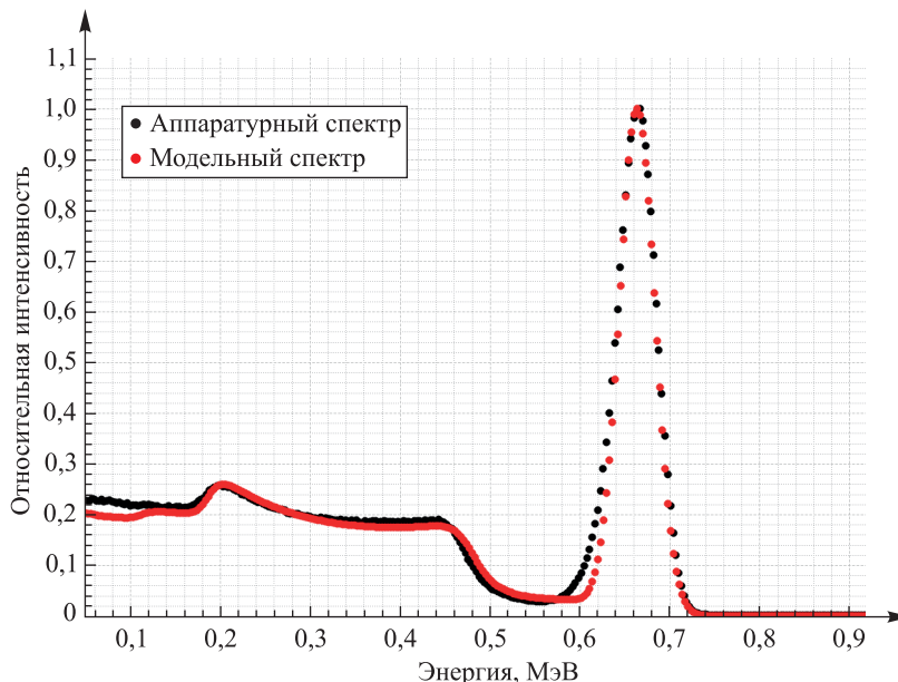
Рис. 2. Сравнение аппаратного и модельного спектров для радионуклида ^{137}\text{Cs}
