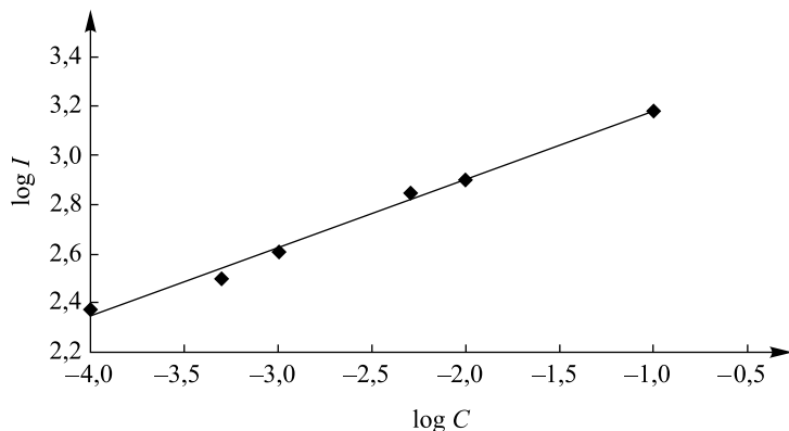
Рис. 1. Градуировочный график для определения концентрации кальция
