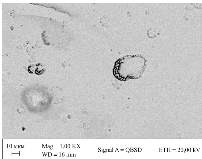
Рис. 3. РЭМ-изображение поверхности пленки CdTe на шлифованной (а), полированной (б) подложках кремния, а также CdTe (в) Fig. 3. REM image of the CdTe film surface on the grinded (a) and polished (b) silicon substrates and on the CdTe substrate (c)
