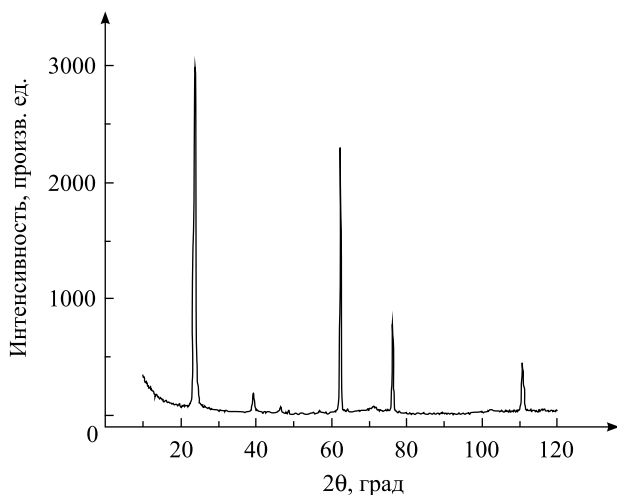
Рис. 4. Рентгенограмма пленки CdTe на подложке из этого же материала ( 2\theta – угол между плоскостью пленки и рентгеновским излучением)
