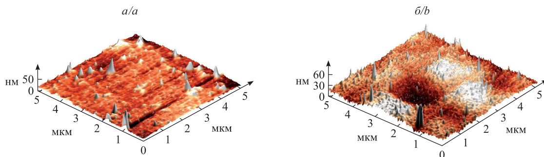
Рис. 2. Трехмерное изображение АСМ-поверхности подложки CdTe (а) и выращенной на ней пленки CdTe (б)
