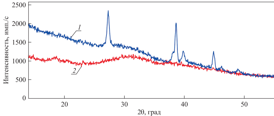
Рис. 3. Дифрактограммы черного (1) и белого (2) порошков
