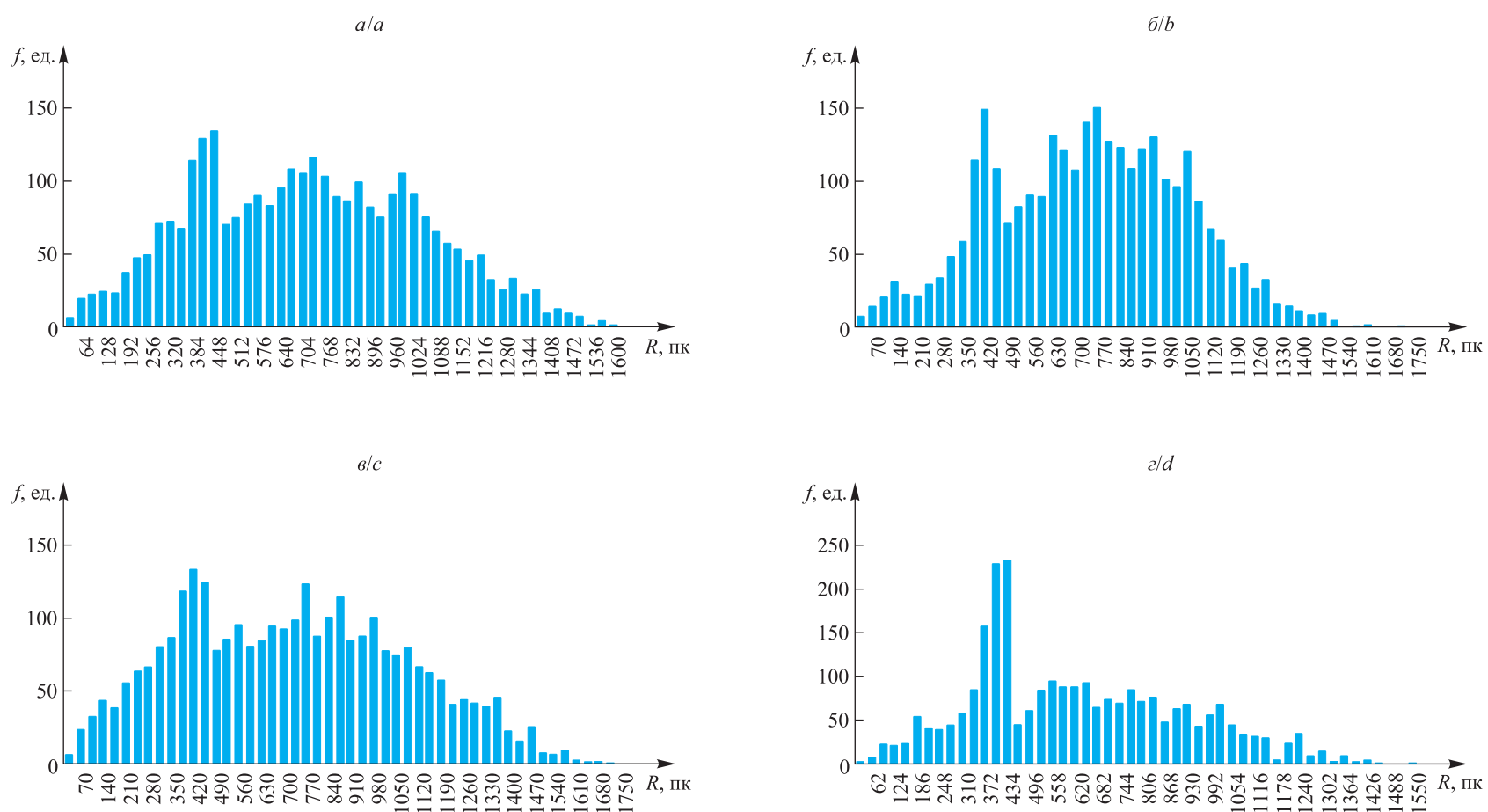
Рис. 1. Гистограммы распределения длин отрезков, соединяющих центры совпадающих областей, построенные с помощью различных детекторов и вычислителей дескрипторов: a – BRISK; б – ORB; в – SURF; г – комбинация методов ORB и FREAK
