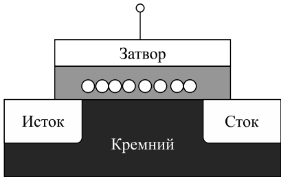
Рис. 1. Транзистор с нанокристаллами. Источник: [3]
