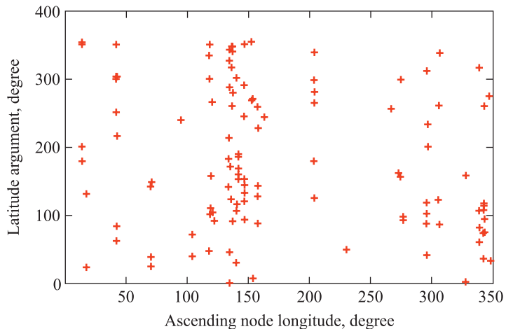
Fig. 1. The dependence of the latitude argument on the ascending node longitude for the Spire Global nanosatellite constellation
