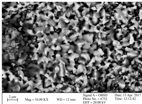
Рис. 2. СЭМ-изображения образцов \text{ZnO} (а), \text{ZnO}_{(90)}\text{FeO}_{(10)-2} (б) и \text{ZnO}_{(90)}\text{Fe}_2\text{O}_{3(10)-2} (в)
