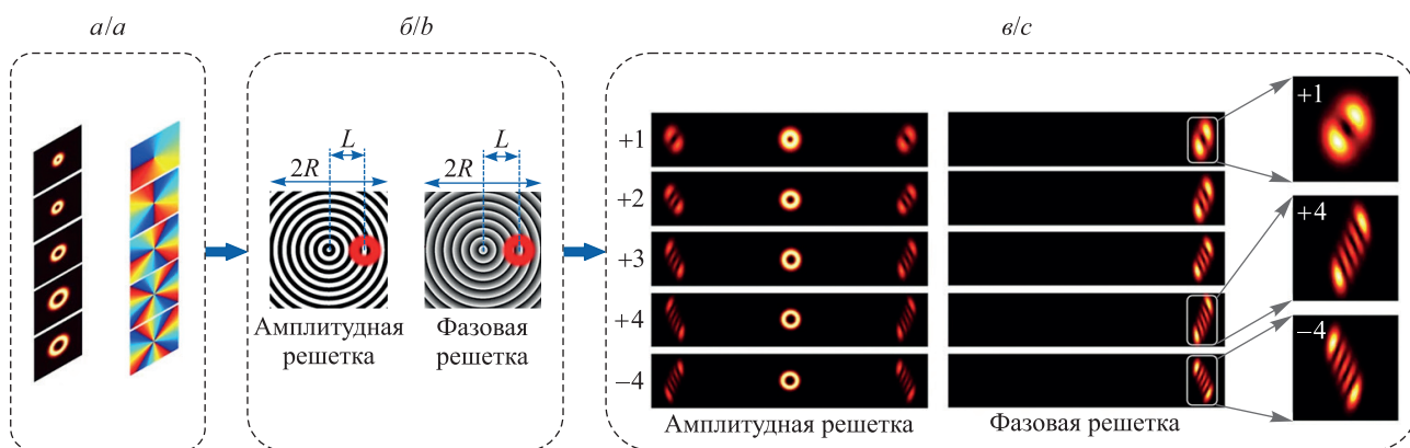
Рис. 10. Принцип измерения момента импульса с помощью кольцевых решеток: а – вихревые (вортксные) пучки; б – кольцевые решетки; в – дифракционные картины. Источник: [18]
