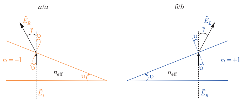
Рис. 8. Оптические схемы модели эквивалентной призмы для левоциркулярно поляризованного (а) и правоициркулярно поляризованного (б) света, нормально падающего на поляризационную дифракционную ЖК-решетку
