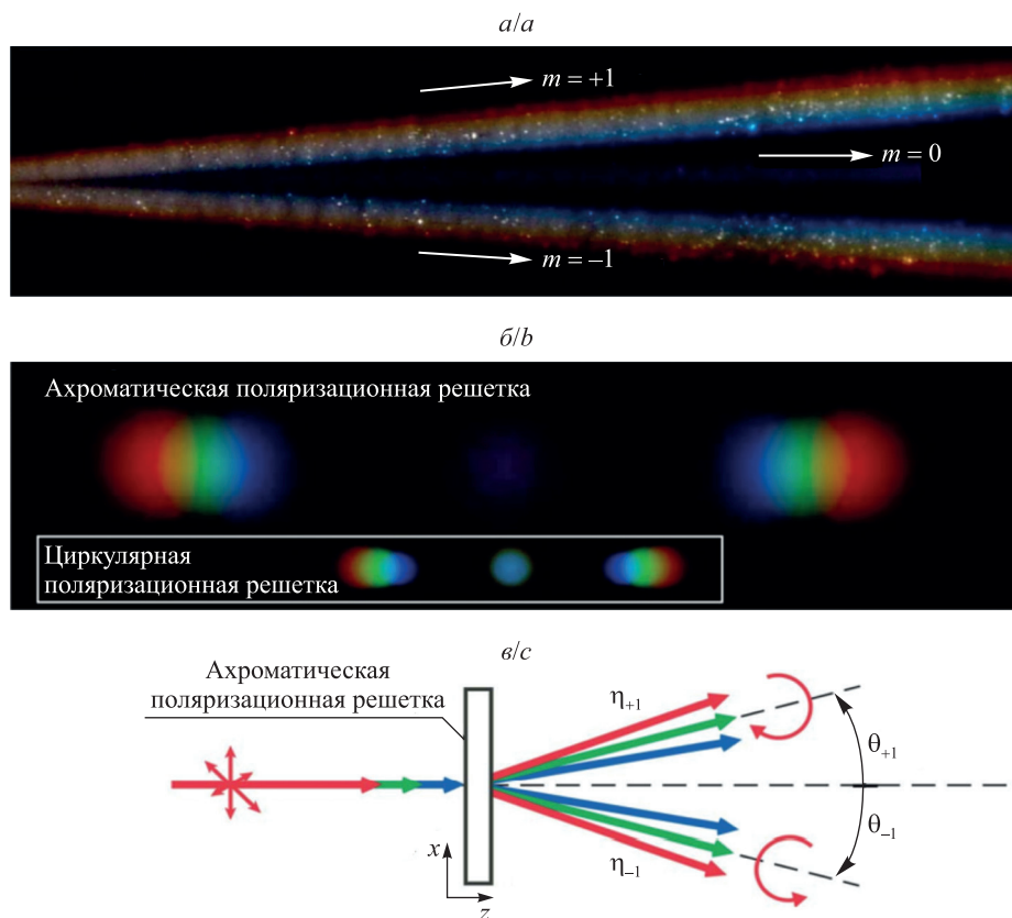
Рис. 5. Фотографии дифракции неполяризованного света белого светодиода на ахроматической поляризационной решетке ( a – вид сверху (при пересечении белой карты); б – вид картины на экране). Оптическая схема дифракции (появляются только порядки m = \pm 1 ) ( в ).
