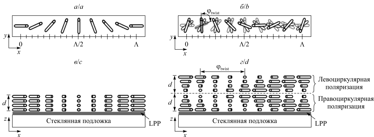
Рис. 4. Базовая геометрия поляризационной решетки ( a – вид сверху; в – вид сбоку). Ахроматическая поляризационная решетка с двумя хиральными слоями ЖК с разным знаком закрутки ( б – вид сверху; г – вид сбоку).
