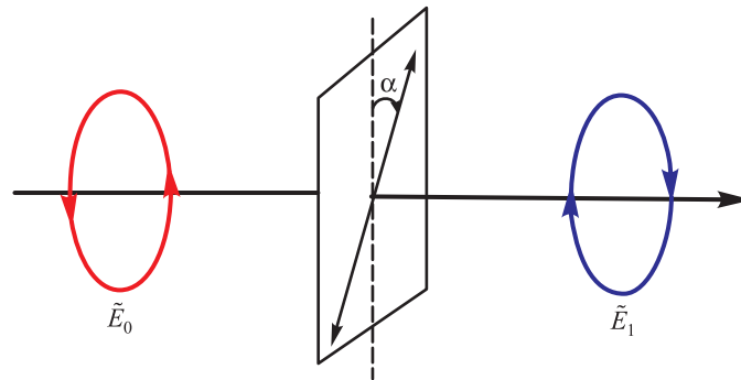
Рис. 3. Нормальное прохождение циркулярно поляризованного света \vec{E}_0 через полуволновую фазовую пластину, повернутую под некоторым углом \alpha
