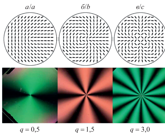
Рис. 14. Примеры картин ЖК с разными топологическими зарядами ( a - 0,5 ; б - 1,5 ; в - 3,0 ) и фотографии соответствующих образцов, помещенных между скрещенными поляризаторами.
