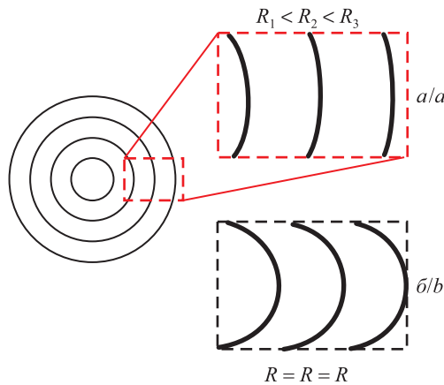
Рис. 12. Схематические изображения кольцевой решетки (a) и решетки с равноотстоящими дугами (b) Fig. 12. Schemes of the annular grating (a) and the grating with equally spaced arcs (b)
