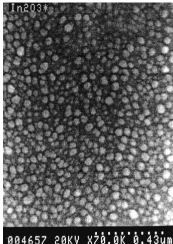
Рис. 1. СЭМ-изображение пленок In 2 O 3 на слюде (а) и распределение их частиц по размерам (б)
