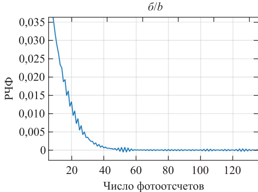
Рис. 3. График действительных значений выражения под экспонентой в ПФ (18) при T = 1,1 \cdot 10^{-4} с (а) и результирующее РЧФ при N_{2MN} = 1 (б)
