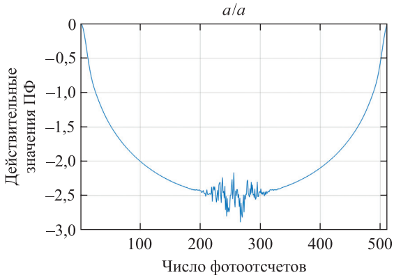
Рис. 3. График действительных значений выражения под экспонентой в ПФ (18) при T = 1,1 \cdot 10^{-4} с (а) и результирующее РЧФ при N_{2MN} = 1 (б)
