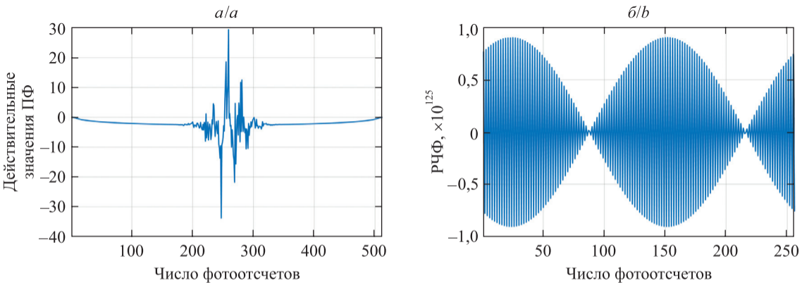
Рис. 4. График действительных значений выражения под экспонентой в ПФ (18) при T = 1,2 \cdot 10^{-4} с ( а ) и результирующее РЧФ ( б )
