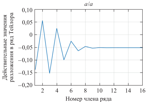
Рис. 5. Вид действительной компоненты в разложении в ряд Тейлора для случаев, рассмотренных на рис. 2 (корректное вычисление РЧФ) (а) и рис. 4 (проблемы с вычислением РЧФ) (б)
