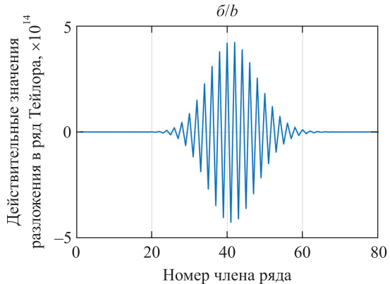
Рис. 5. Вид действительной компоненты в разложении в ряд Тейлора для случаев, рассмотренных на рис. 2 (корректное вычисление РЧФ) (а) и рис. 4 (проблемы с вычислением РЧФ) (б)
