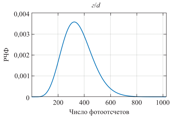
Рис. 6. Графики значений подэкспоненциального выражения в ПФ ( a, v ) и результирующего РЧФ ( b, z ) для случаев, рассмотренных на рис. 2 ( a, b ) и рис. 4 ( v, z ) Fig. 6. Graphs of the values of the expression under the exponent in generating function ( a, v ) and the resulting PCD ( b, z ) for the cases considered in fig. 2 ( a, b ) and fig. 4 ( c, d )
