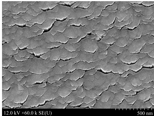
Рис. 4. СЭМ-микрофотографии поверхности ( а ) и скола ( б ) покрытия TiAlCN, сформированного на кремниевой подложке в режиме 1 с соотношением парциальных давлений азота и ацетилена P_{N_2} : P_{C_2H_2} = 1 : 1 Fig. 4. SEM micrographs of the surface ( a ) and cleavage ( b ) of TiAlCN coating formed on silicon substrates in regime 1 with the ratio of partial pressures of nitrogen and acetylene P_{N_2} : P_{C_2H_2} = 1 : 1
