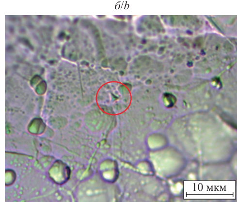
Рис. 8. Кривые нагрузки-разгрузки ( a ) и фотография отпечатка индентора ( б ) для покрытия TiAlCN, сформированного в режиме 2 с соотношением парциальных давлений азота и ацетилена P_{N_2} : P_{C_2H_2} = 2 : 1 ( H – нанотвердость; E – модуль Юнга; S – жесткость; F_{\max} – максимальная нагрузка; h_{\max} – максимальная глубина проникновения индентора)
