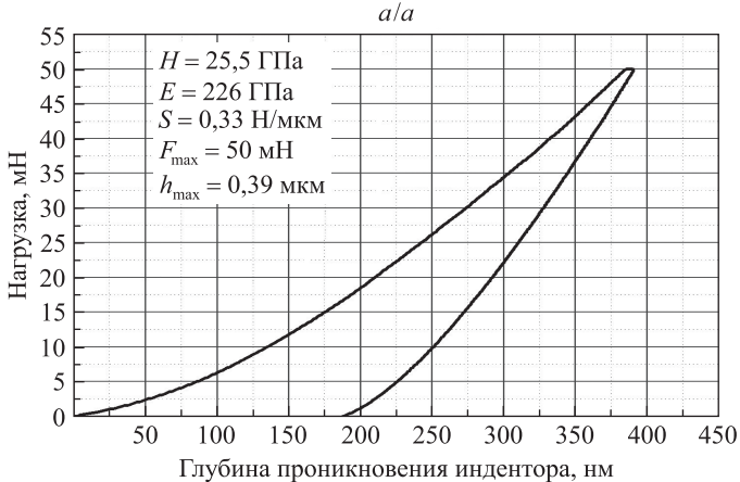
Рис. 8. Кривые нагрузки-разгрузки ( a ) и фотография отпечатка индентора ( б ) для покрытия TiAlCN, сформированного в режиме 2 с соотношением парциальных давлений азота и ацетилена P_{N_2} : P_{C_2H_2} = 2 : 1 ( H – нанотвердость; E – модуль Юнга; S – жесткость; F_{\max} – максимальная нагрузка; h_{\max} – максимальная глубина проникновения индентора)
