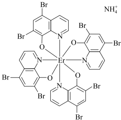
Рис. 2. Формулы комплексов на основе производных хинолина. Источник: [15]
