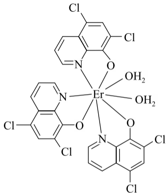
Рис. 2. Формулы комплексов на основе производных хинолина. Источник: [15]
