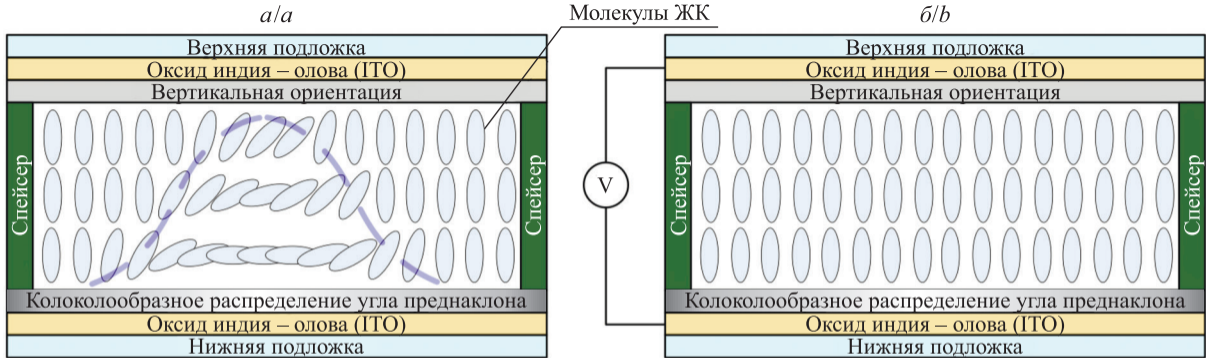
Рис. 1. Схема управляемой ЖК-линзы в плоской ячейке: a – без приложенного напряжения; b – с приложенным напряжением.
