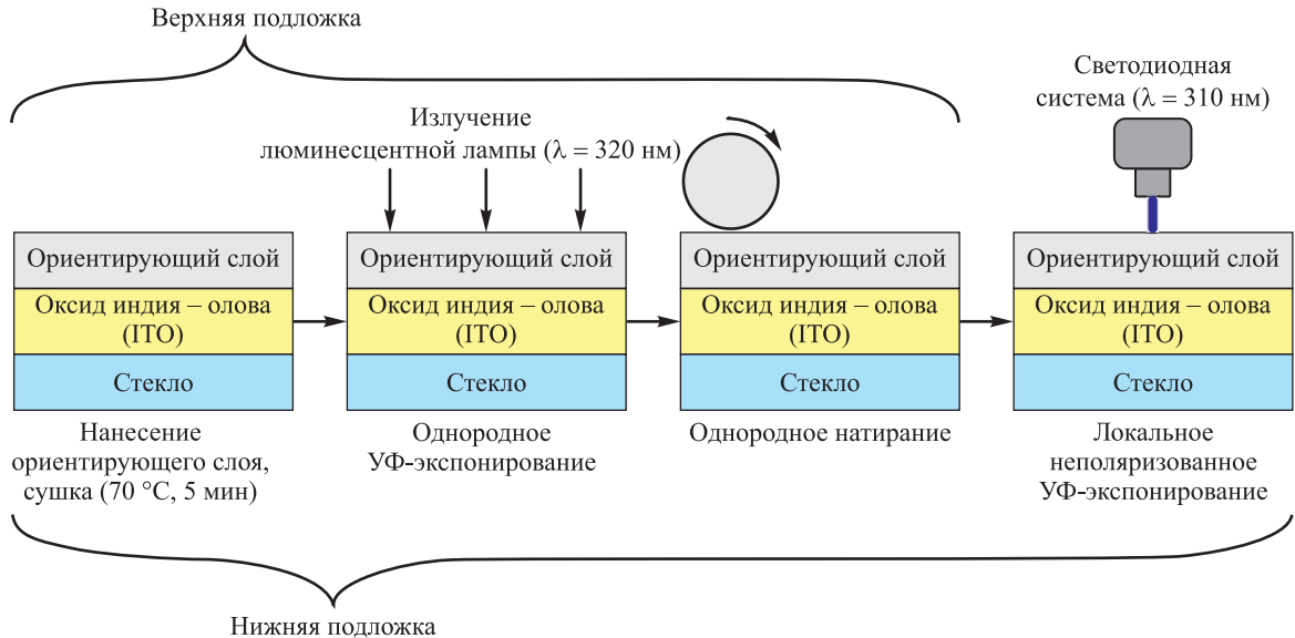
Рис. 2. Схема технологии изготовления ЖК-ячейки для формирования ЖК-линзы методом фотостимулированной ориентации с использованием светодиодной системы ( \lambda = 310 \text{ нм} )
